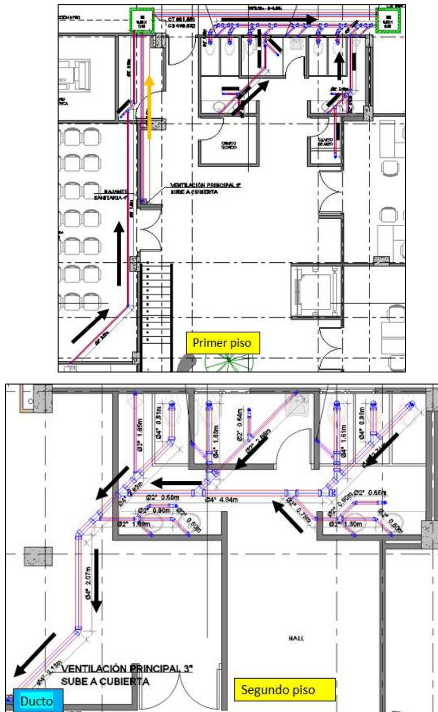
Figura 6-1. Implantación redes sanitarias primer y segundo piso.
