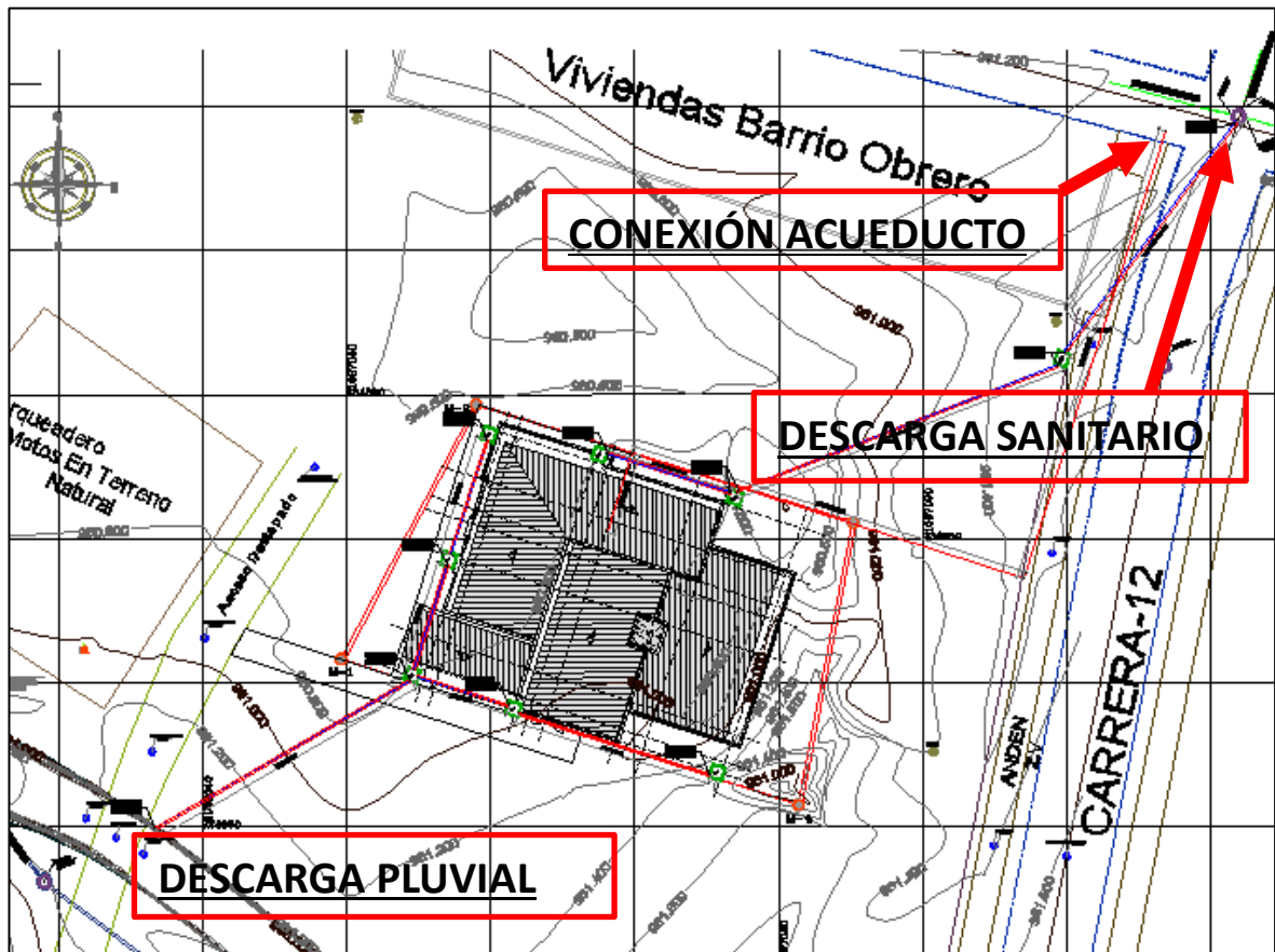
Figura 4-6. Localización abastecimiento y descargas.
