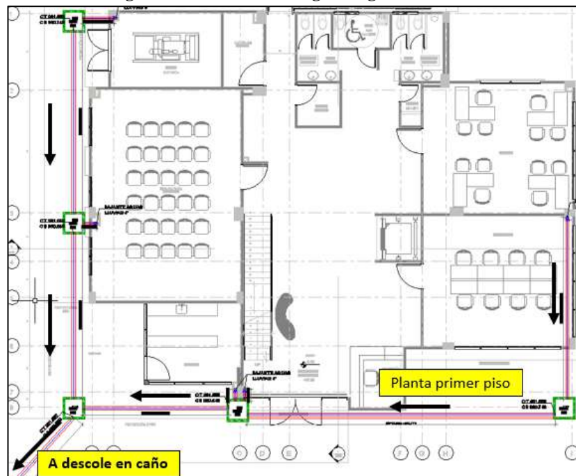
Figura 7-5. Red de descarga de aguas lluvias.
