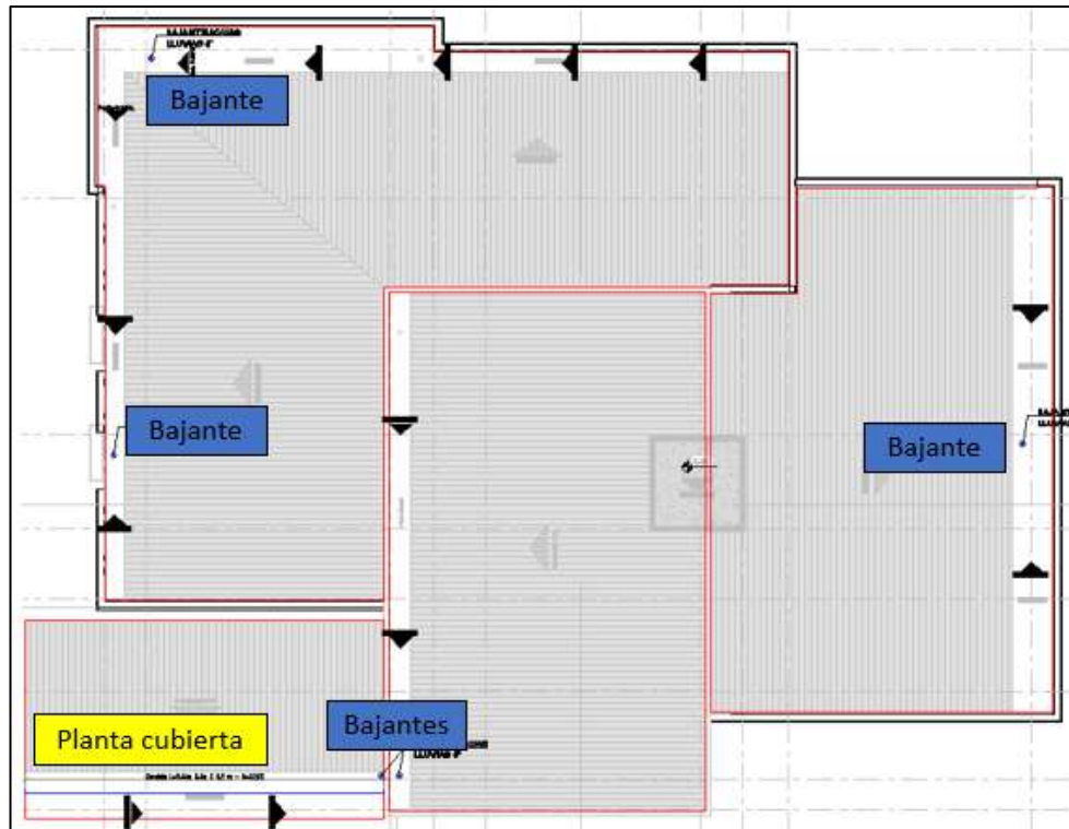
Figura 7-4. Sistema de evacuación y recolección aguas lluvias.
