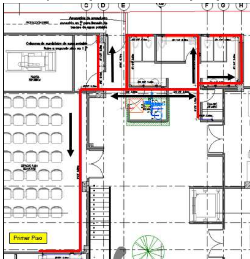
Figura 5-1. Implantación redes hidráulicas primer piso.
