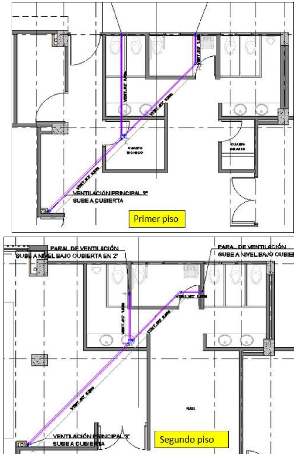
Figura 6-2. Implantación redes ventilación primer y segundo piso.
