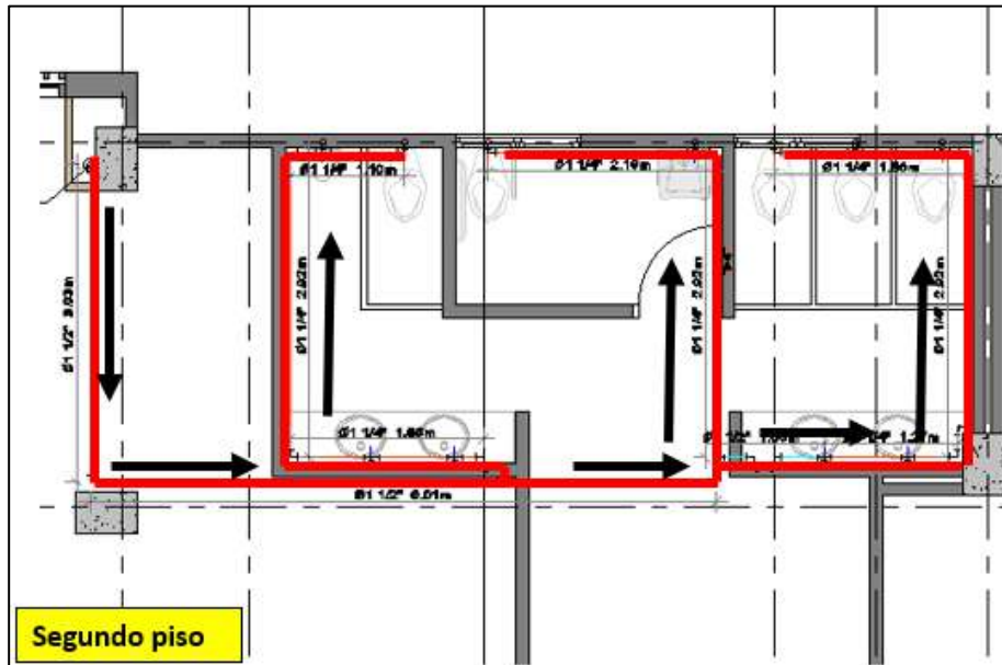
Figura 5-2. Implantación redes hidráulicas segundo piso.
