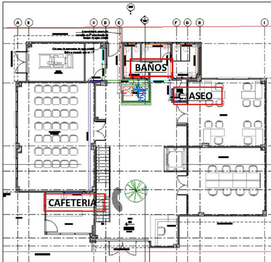
Figura 4-4. Vista en planta primer piso.
