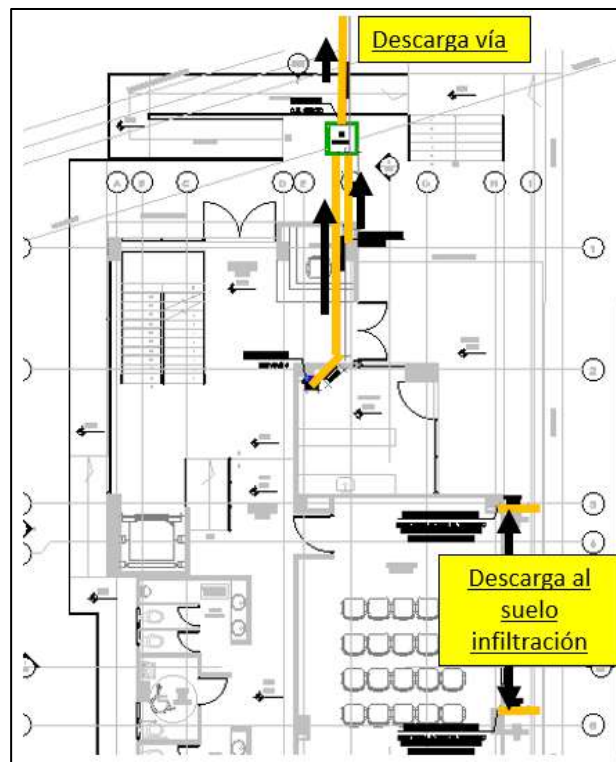
Figura 7. 4. Red de descarga de aguas lluvias.
