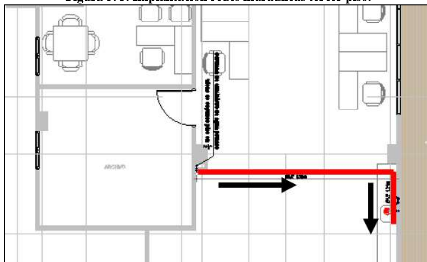
Figura 5. 3. Implantación redes hidráulicas tercer piso.
