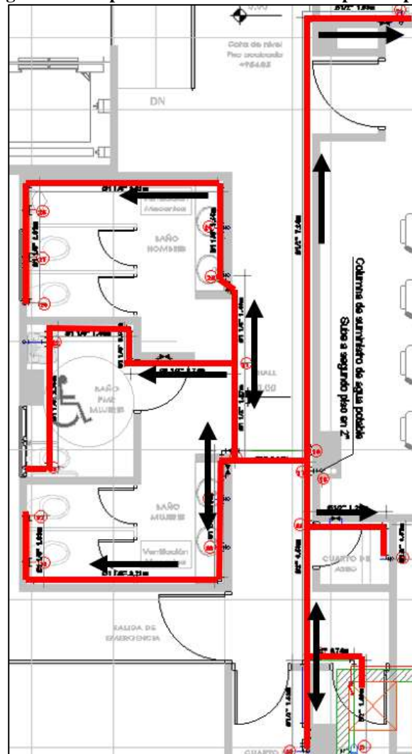
Figura 5. 1. Implantación redes hidráulicas primer piso.
