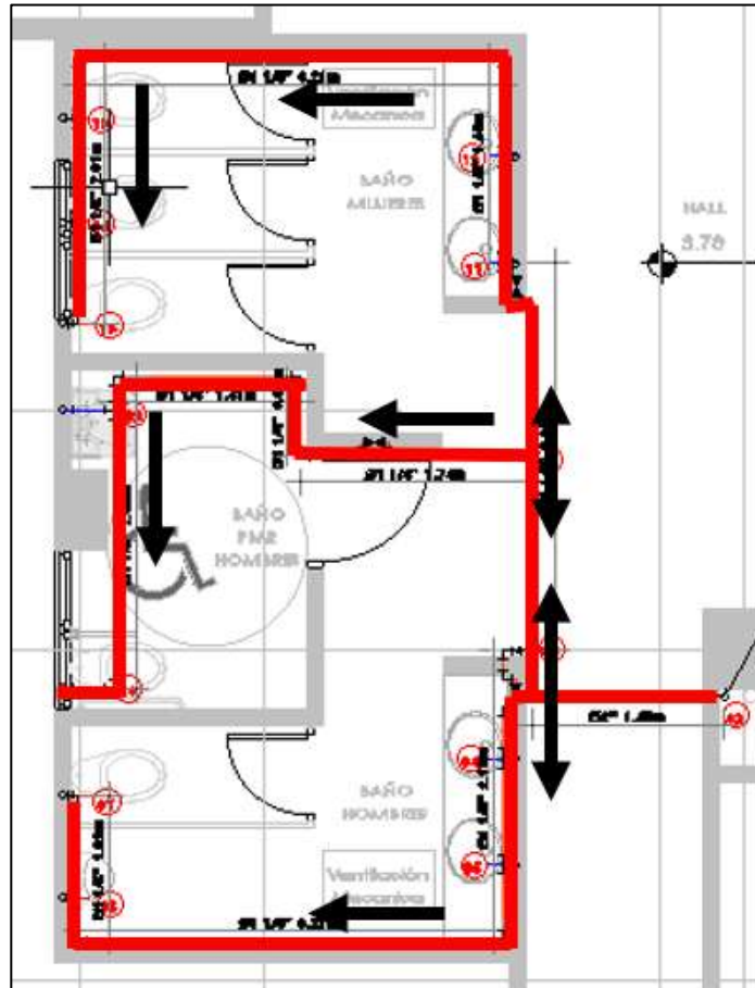
Figura 5. 2. Implantación redes hidráulicas segundo piso.
