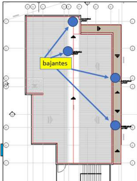
Figura 7. 3. Sistema de evacuación y recolección aguas lluvias.
