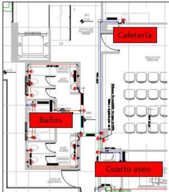
Figura 4. 2. Vista en planta primer piso.
