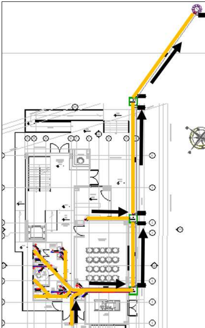
Figura 6. 1. Implantación redes sanitarias primer piso
