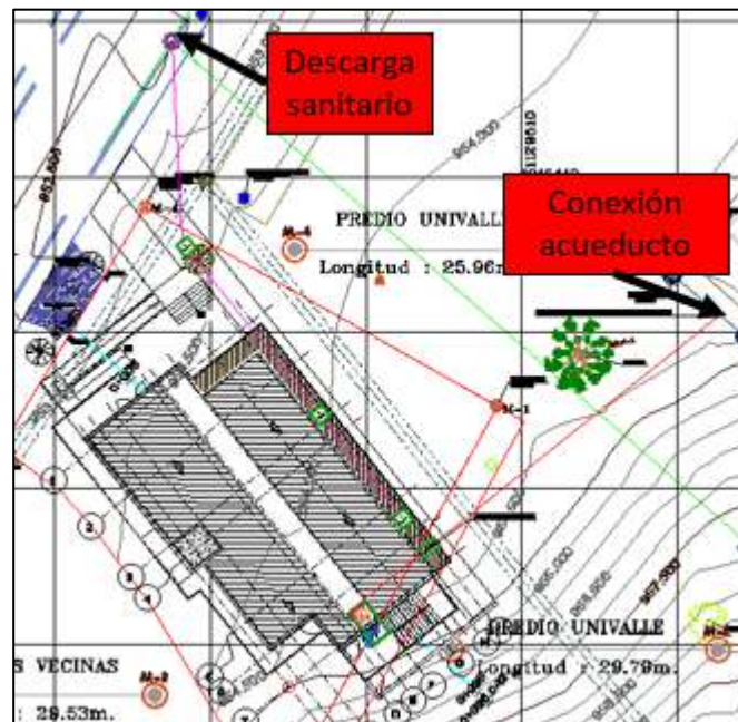
Figura 4. 5. Localización abastecimiento y descargas.
