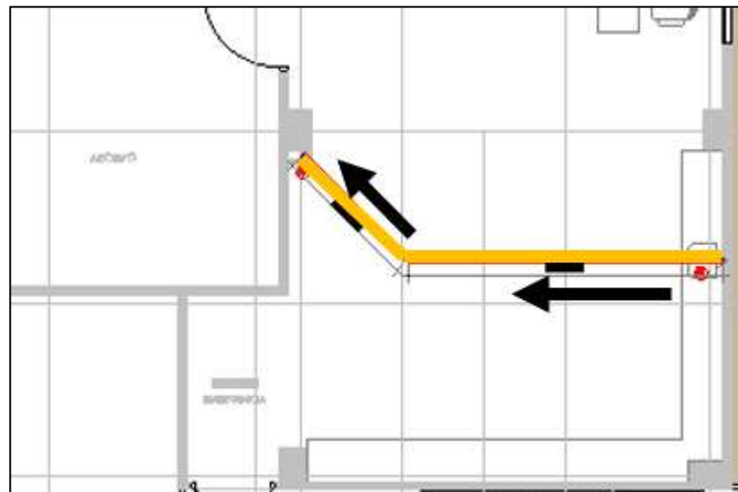
Figura 6. 3. Implantación redes sanitarias tercer piso
