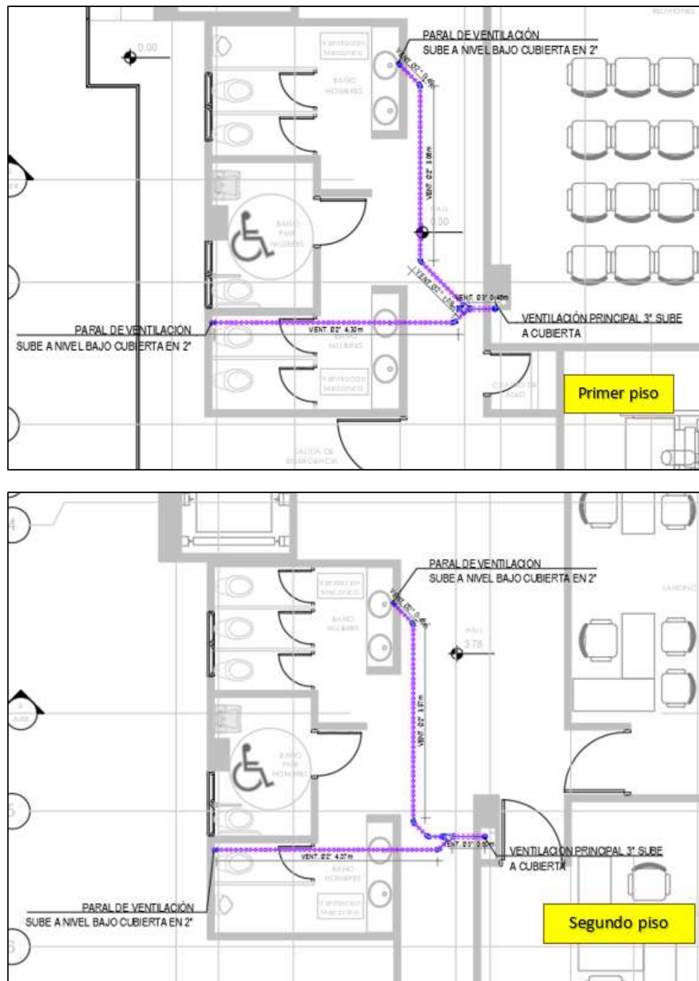
Figura 6. 4. Implantación redes ventilación primer y segundo piso.
