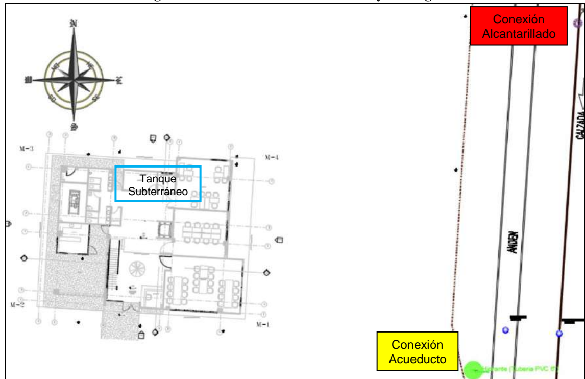
Figura 4-6. Localización abastecimiento y descargas.
