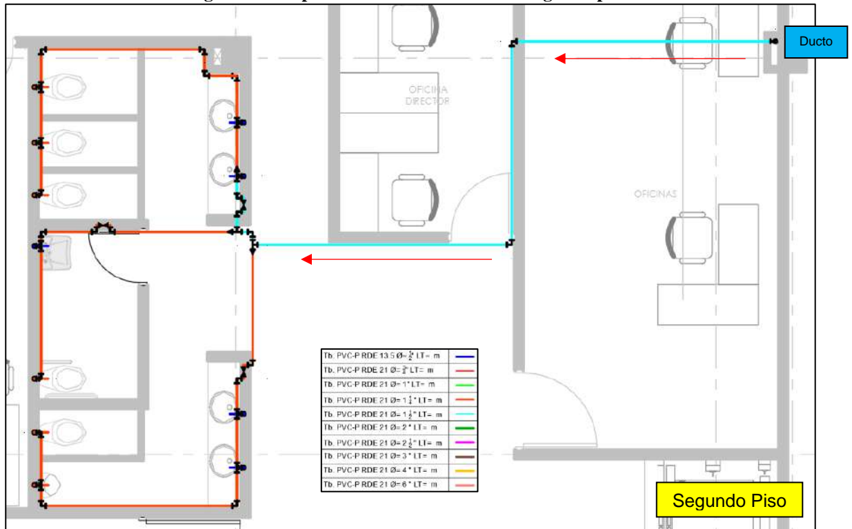
Figura 5-2. Implantación redes hidráulicas segundo piso.
