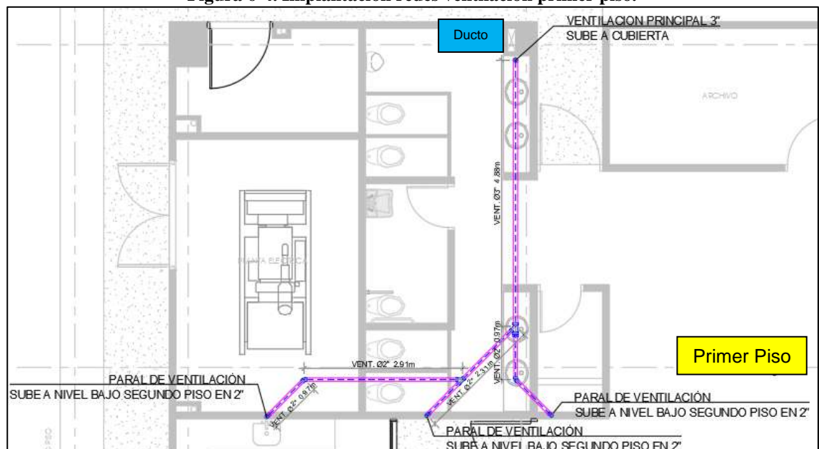
Figura 6-4. Implantación redes ventilación primer piso.
