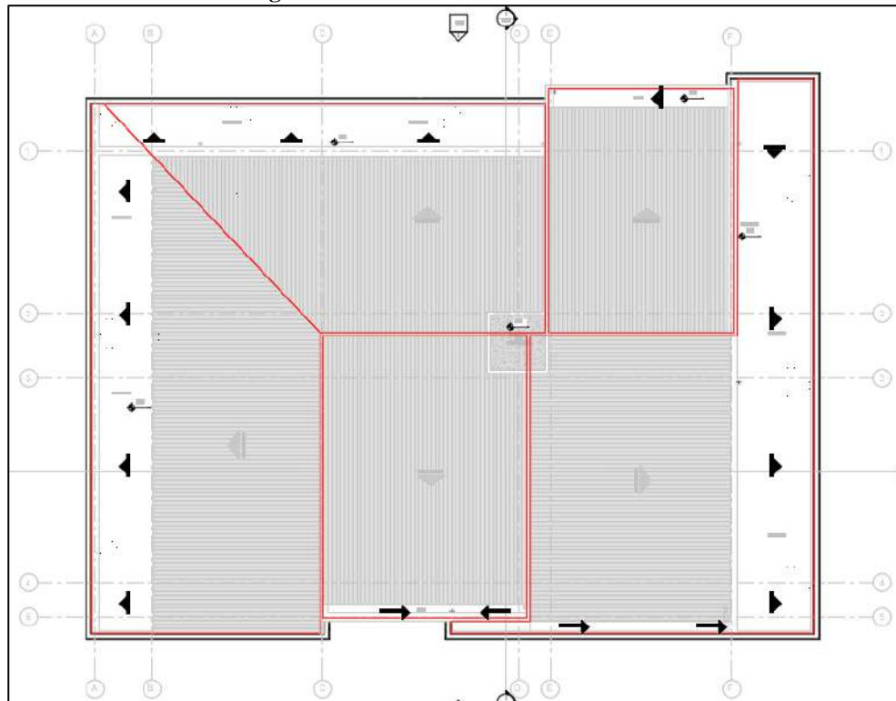
Figura 7-1. Sectorización áreas cubierta.
