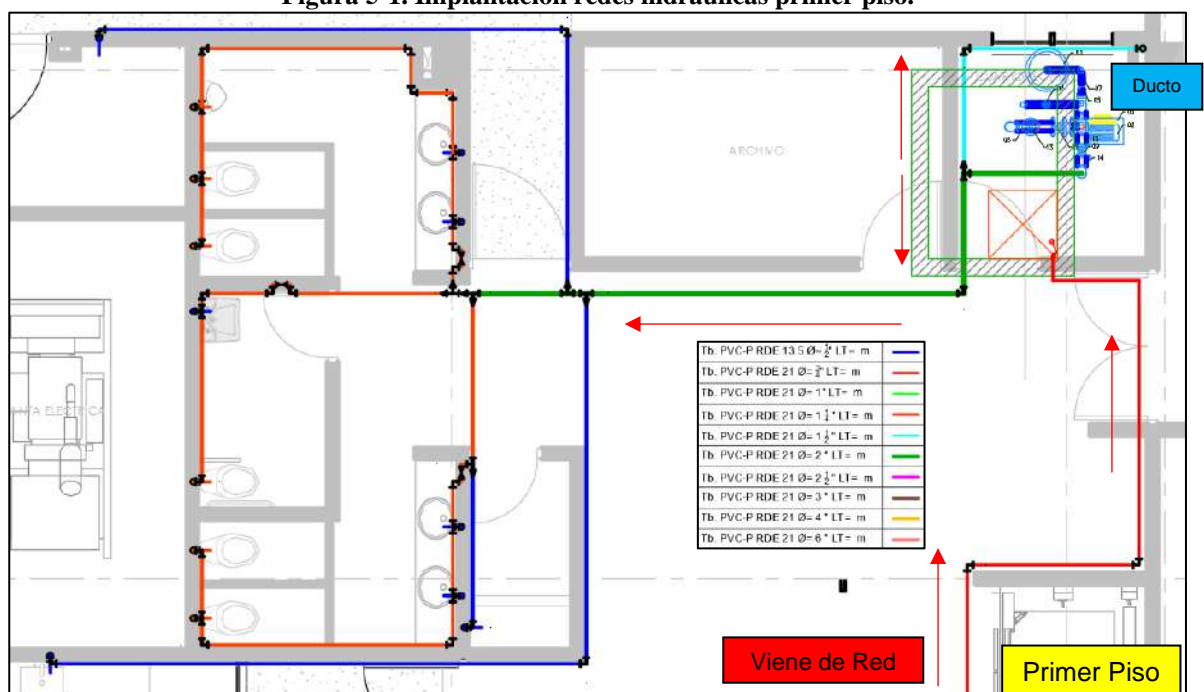
Figura 5-1. Implantación redes hidráulicas primer piso.
