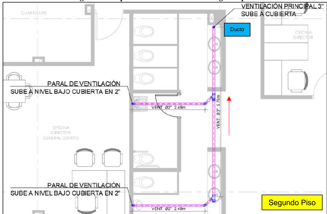
Figura 6-2. Implantación redes ventilación segundo piso.
