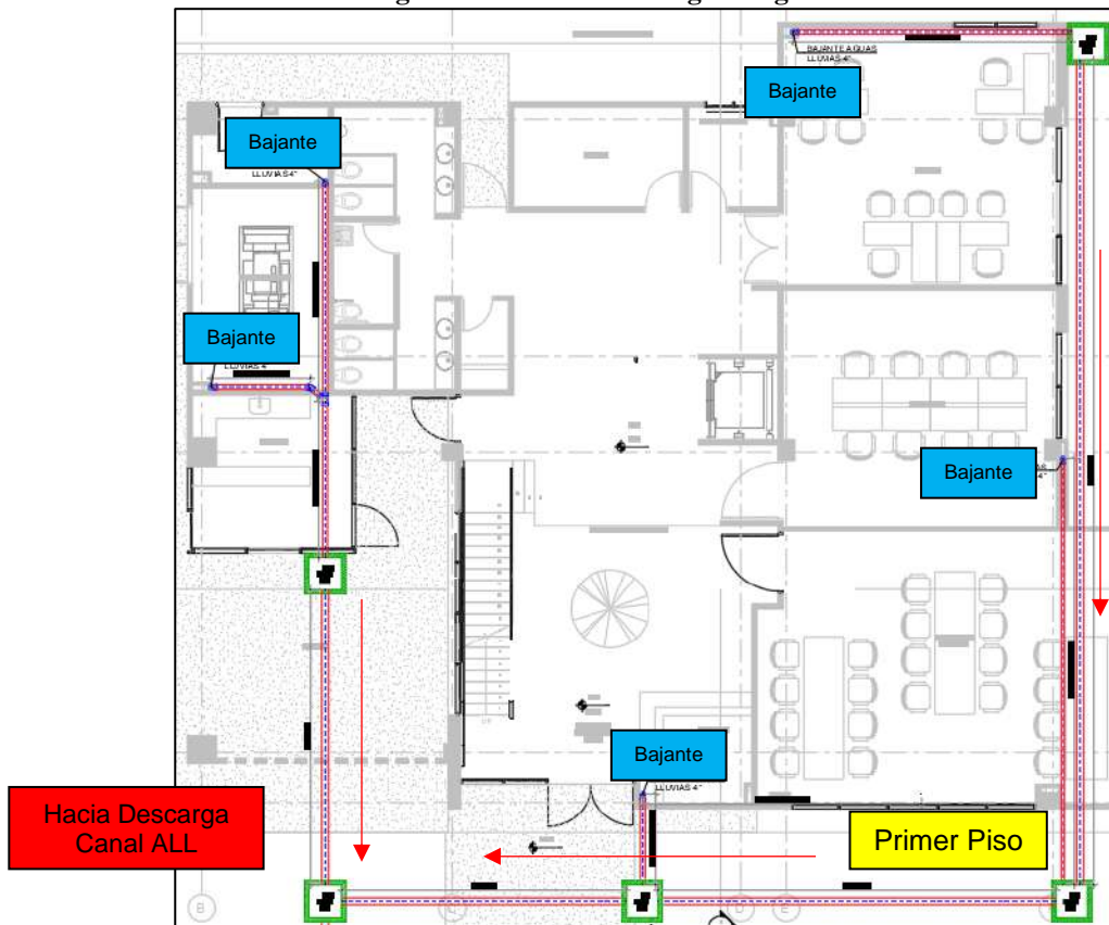
Figura 7-5. Red de descarga de aguas lluvias.
