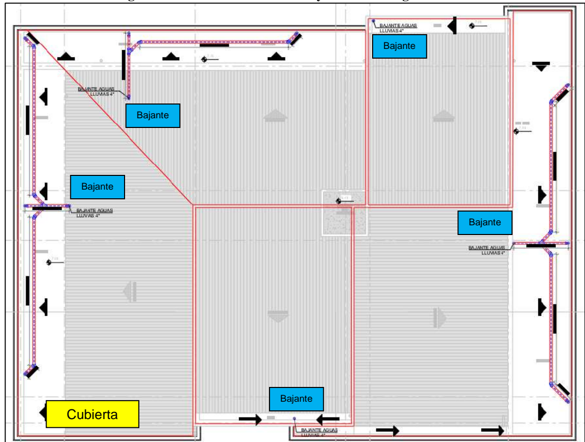
Figura 7-4. Sistema de evacuación y recolección aguas lluvias.
