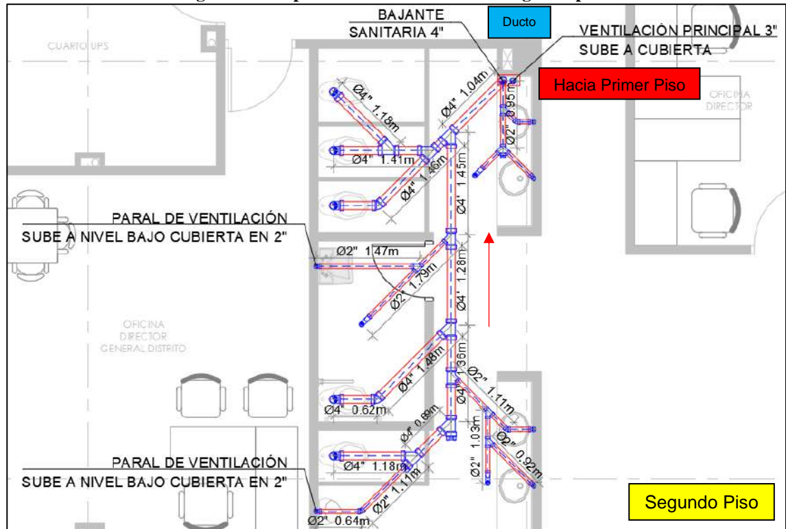
Figura 6-1. Implantación redes sanitarias segundo piso.
