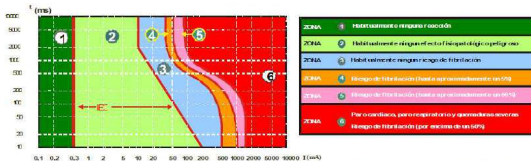
1. Zonas de tiempo/corriente de los efectos de las corrientes alternas de 15 Hz a 100 Hz
