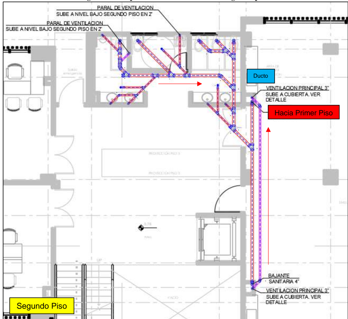
Figura 6-3. Implantación redes sanitarias segundo piso.
