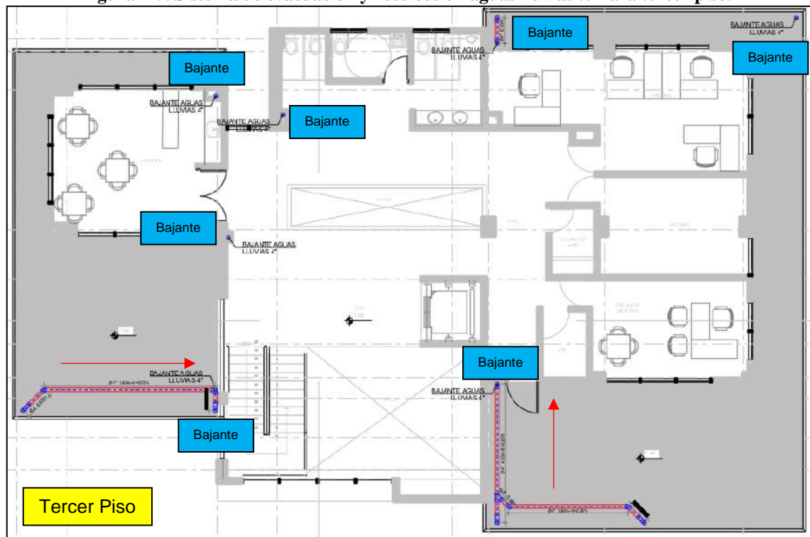
Figura 7-5. Sistema de evacuación y recolección aguas lluvias terraza tercer piso.
