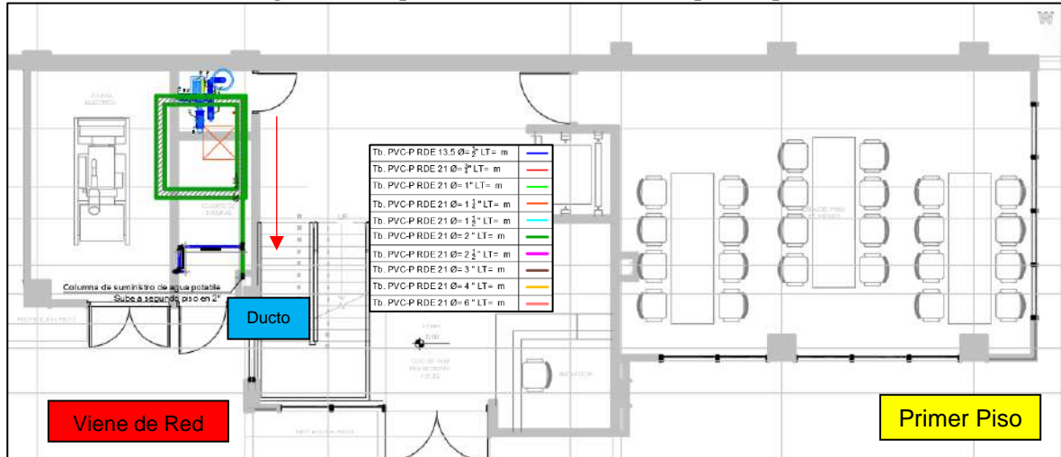
Figura 5-1. Implantación redes hidráulicas primer piso.
