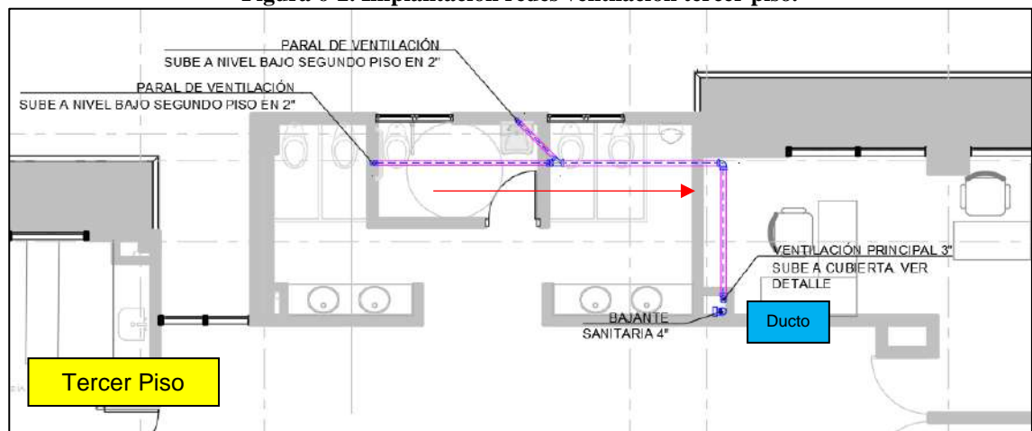
Figura 6-2. Implantación redes ventilación tercer piso.
