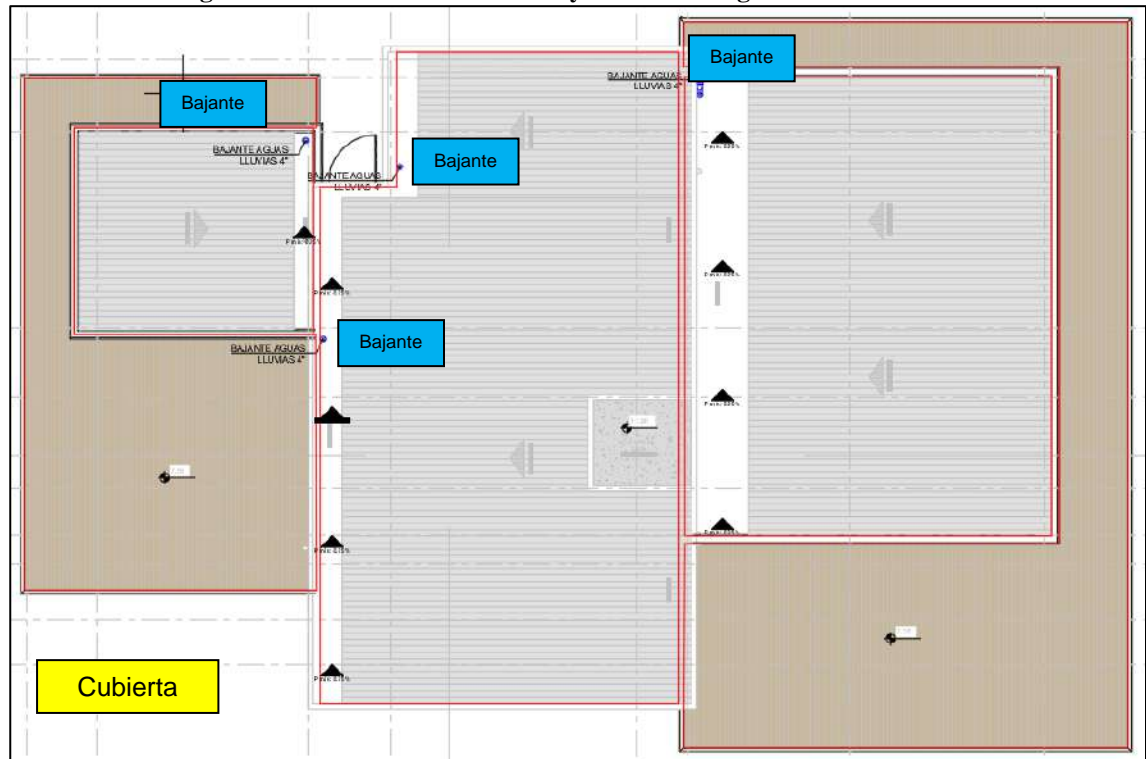
Figura 7-4. Sistema de evacuación y recolección aguas lluvias cubierta.
