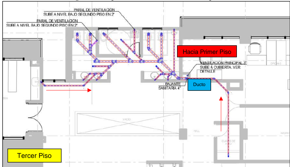
Figura 6-1. Implantación redes sanitarias tercer piso.
