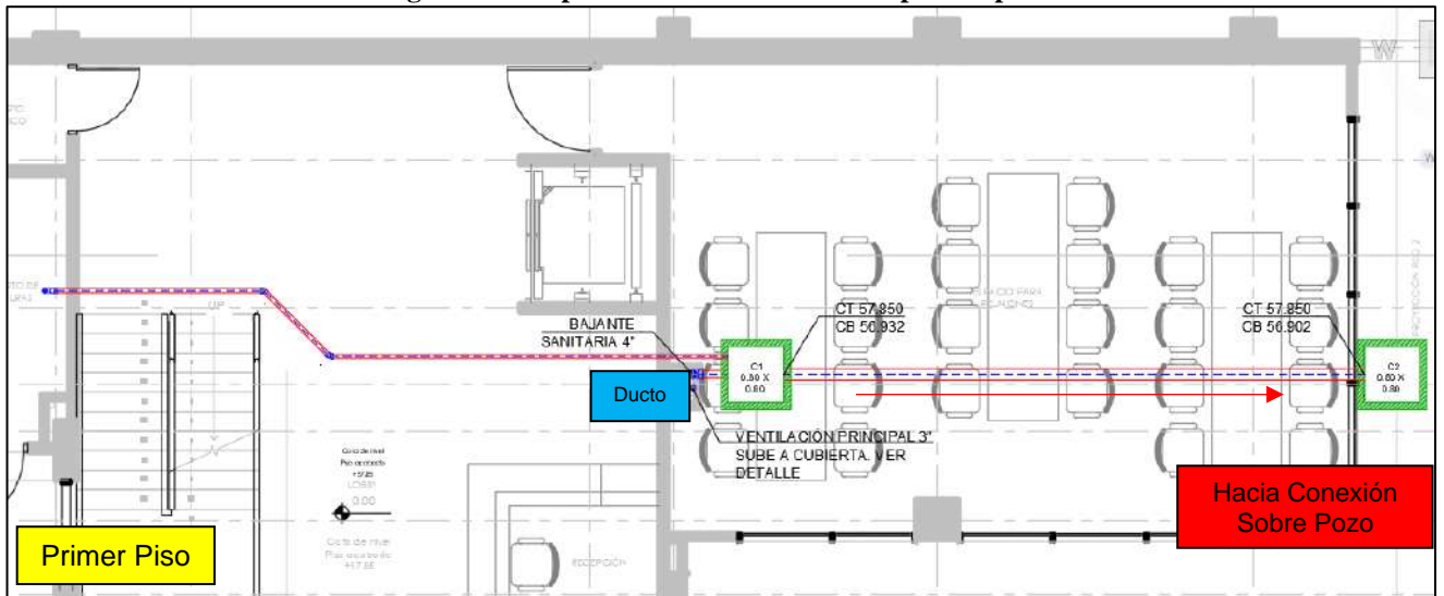
Figura 6-5. Implantación redes sanitarias primer piso.
