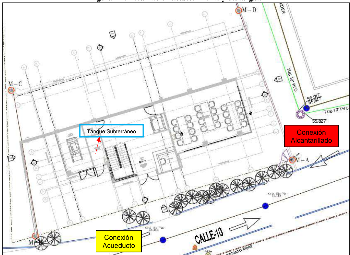
Figura 4-7. Localización abastecimiento y descargas.
