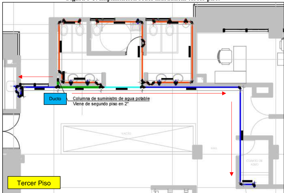
Figura 5-3. Implantación redes hidráulicas tercer piso.
