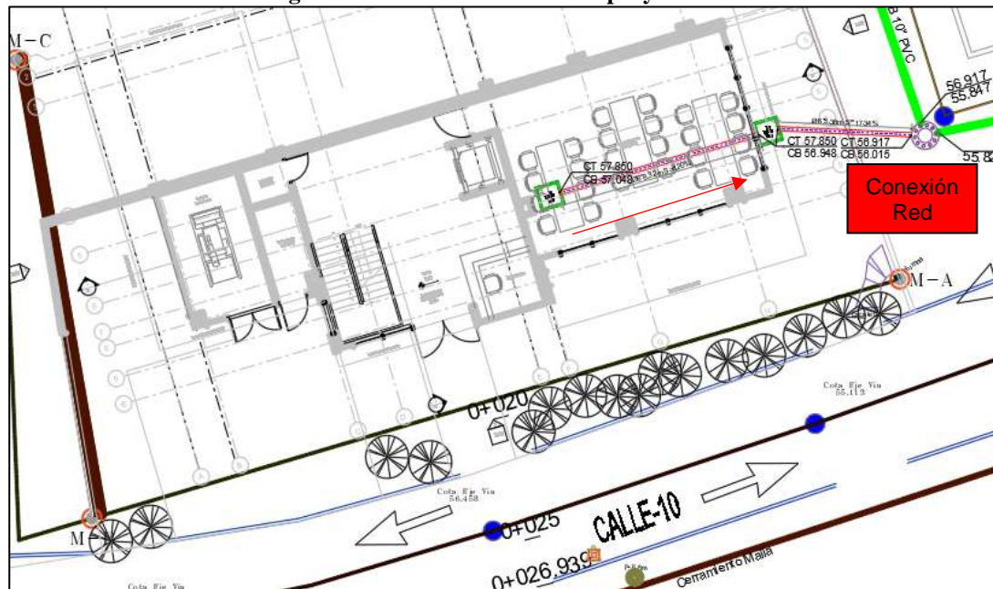
Figura 6-6. Redes alcantarillado proyectadas.
