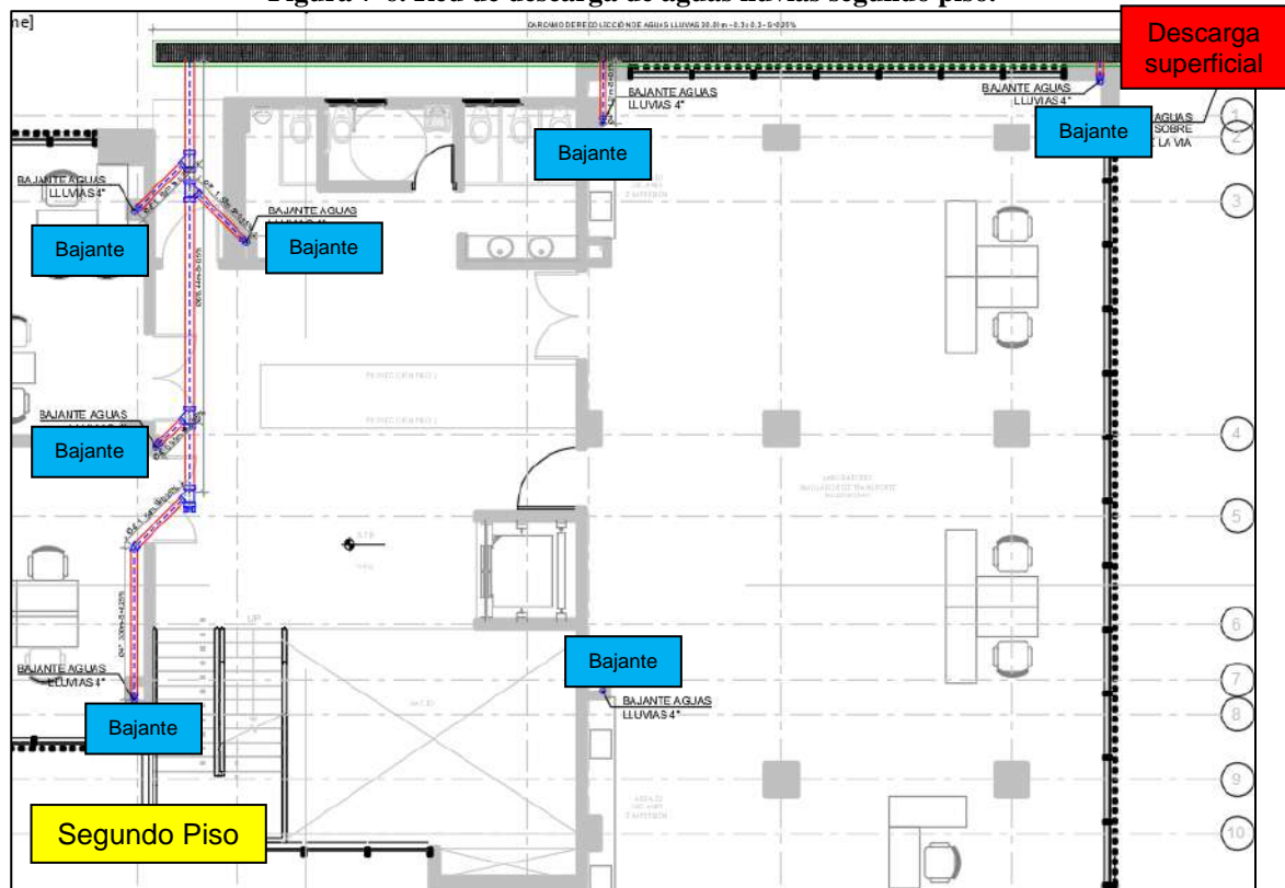
Figura 7-6. Red de descarga de aguas lluvias segundo piso.
