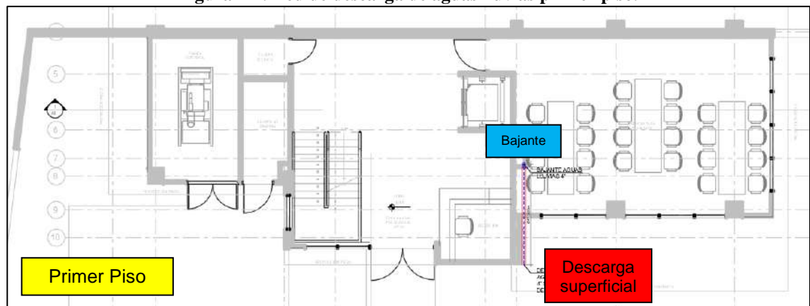
Figura 7-7. Red de descarga de aguas lluvias primer piso.
