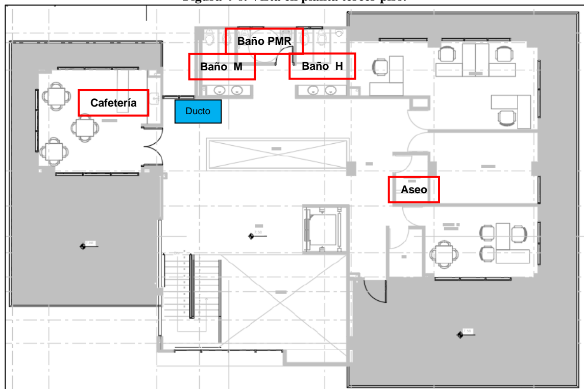
Figura 4-6. Vista en planta tercer piso.
