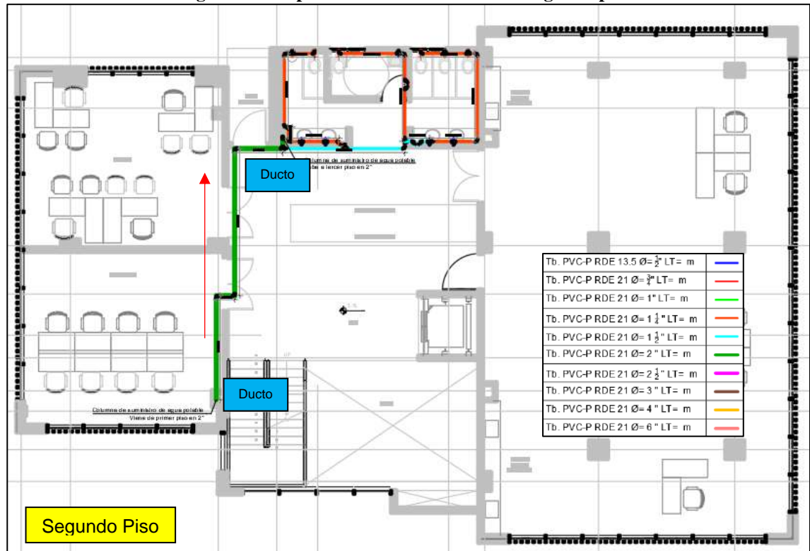
Figura 5-2. Implantación redes hidráulicas segundo piso.
