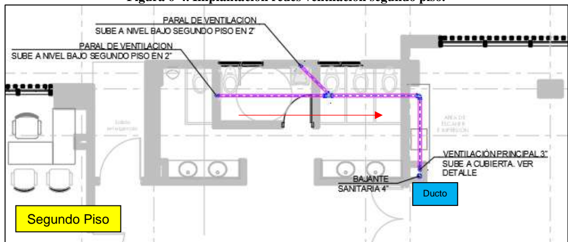
Figura 6-4. Implantación redes ventilación segundo piso.
