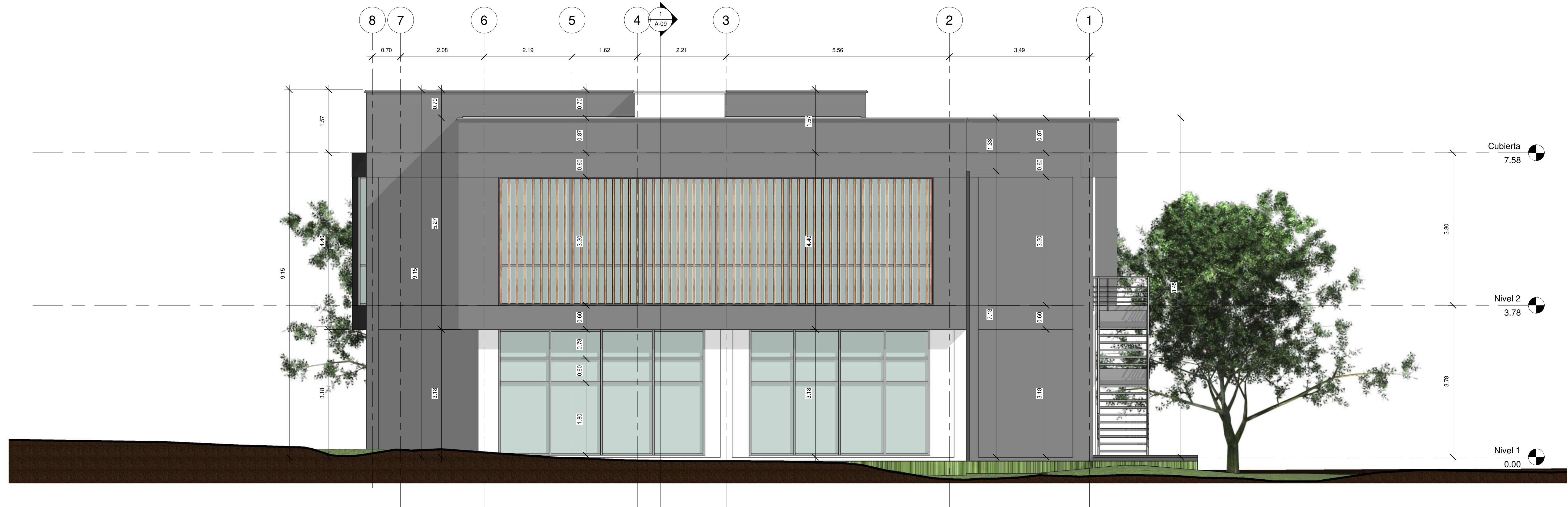
1 Este 1 : 50
