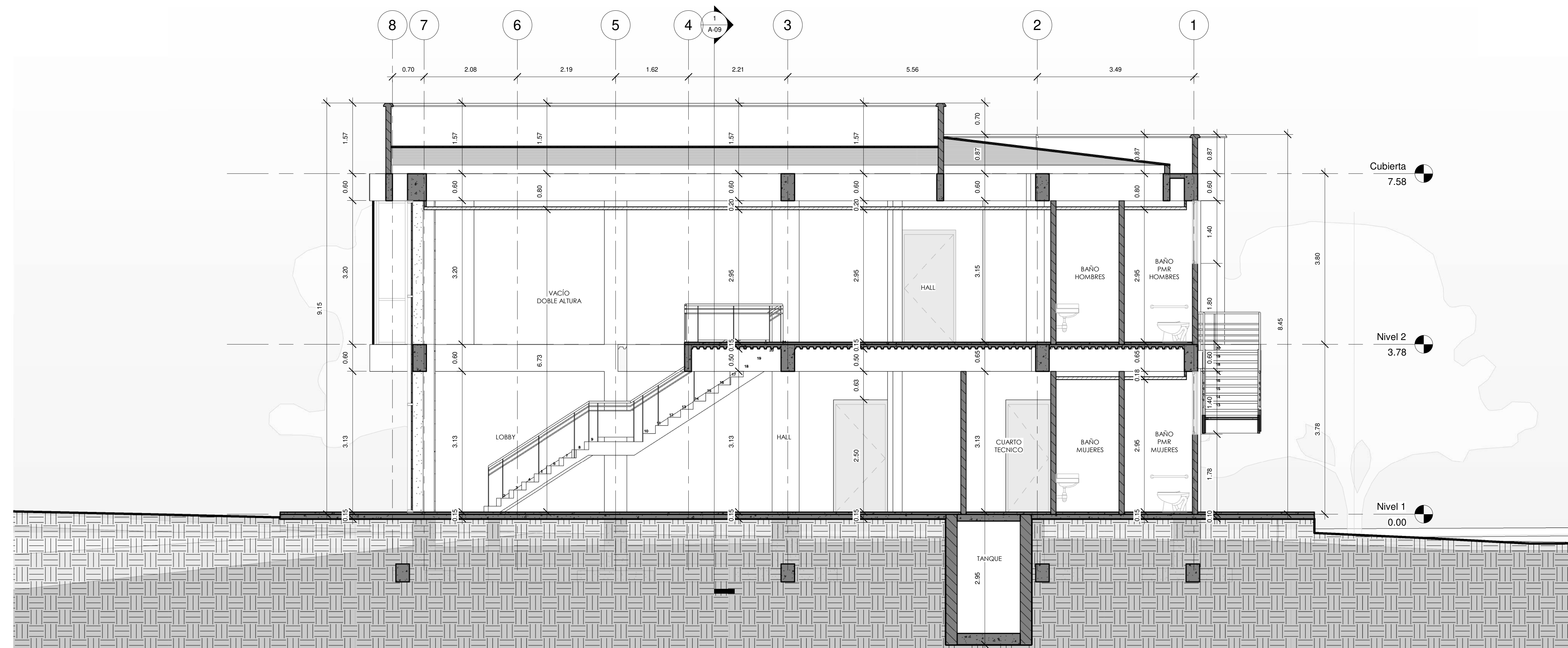
1 Corte Transversal B-B 1 : 50
