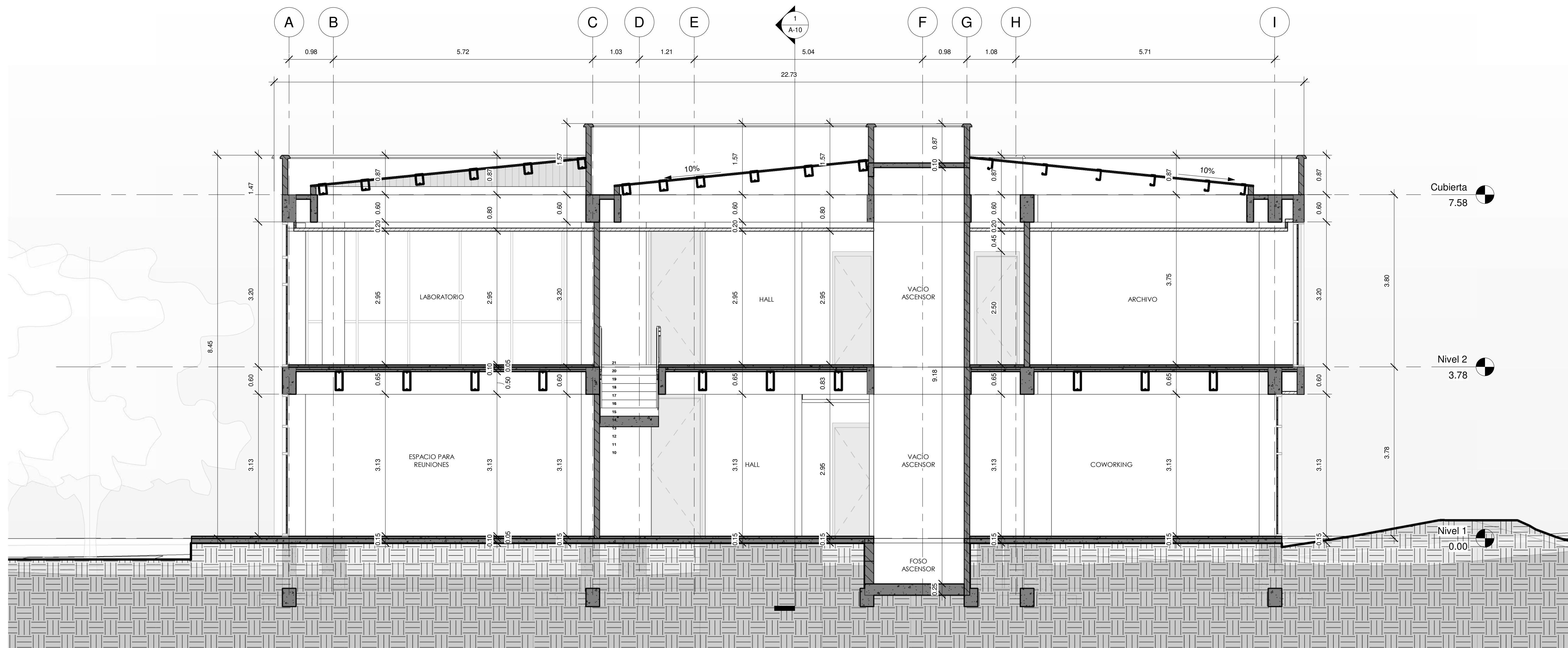
1 Corte Longitudinal A-A 1 : 50
