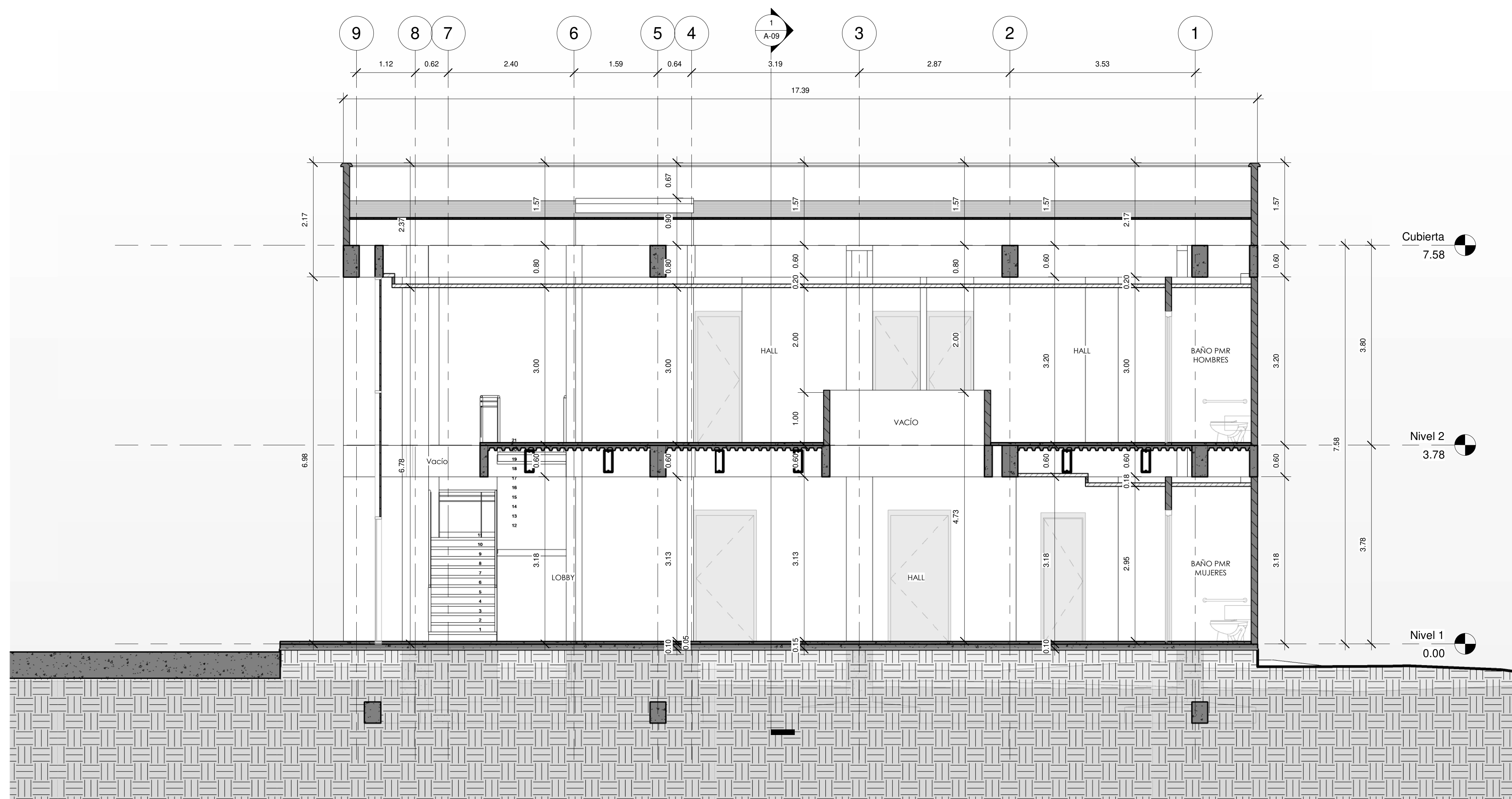
1 Corte transversal B-B 1 : 50
