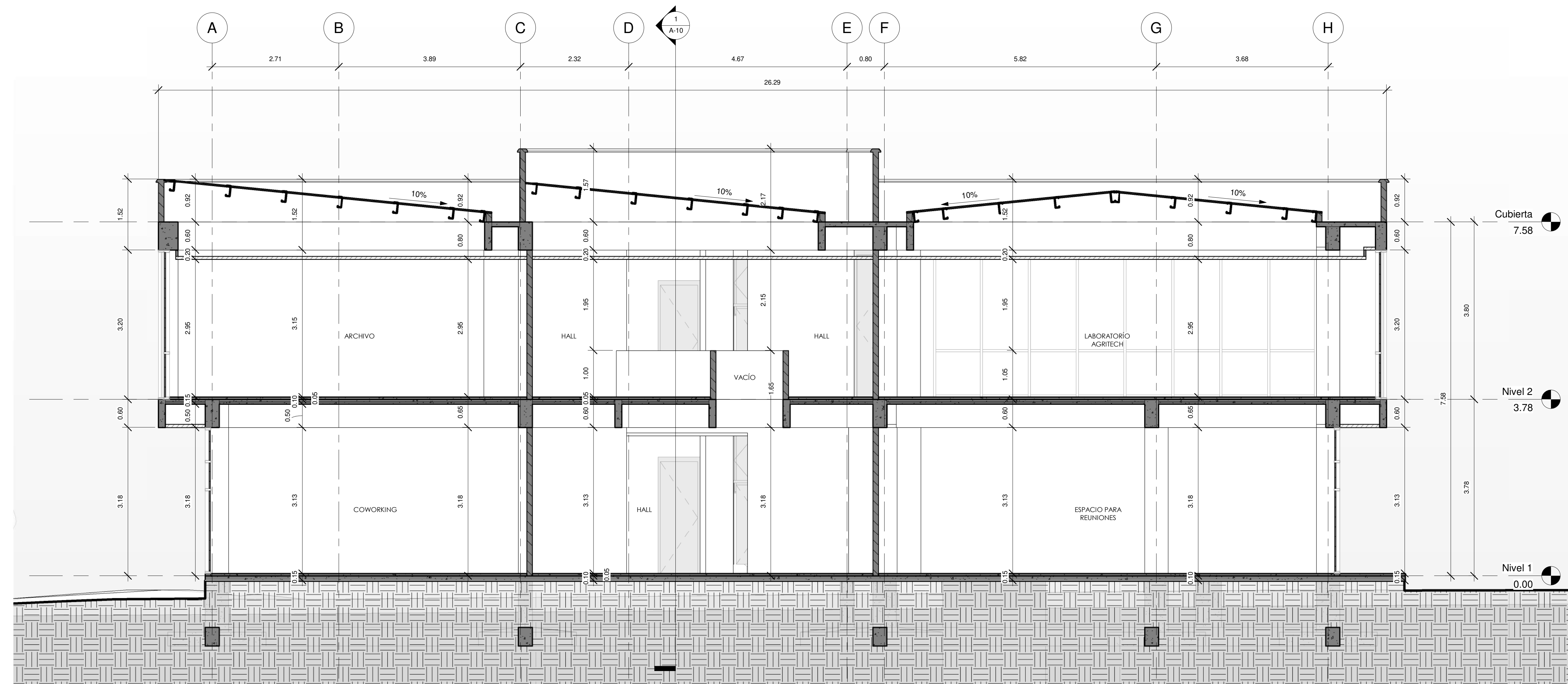
1 Corte Longitudinal A-A 1 : 50
