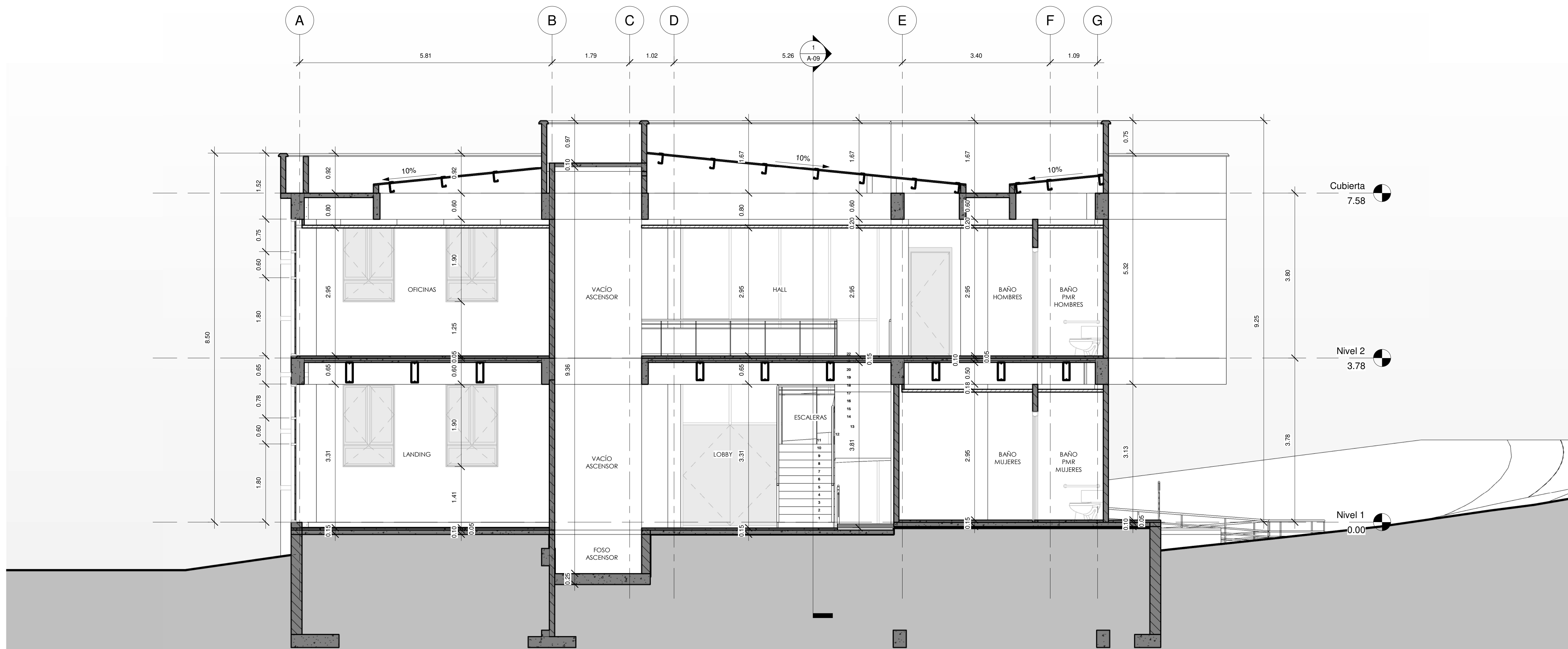
1 Corte Transversal B-B 1 : 50
