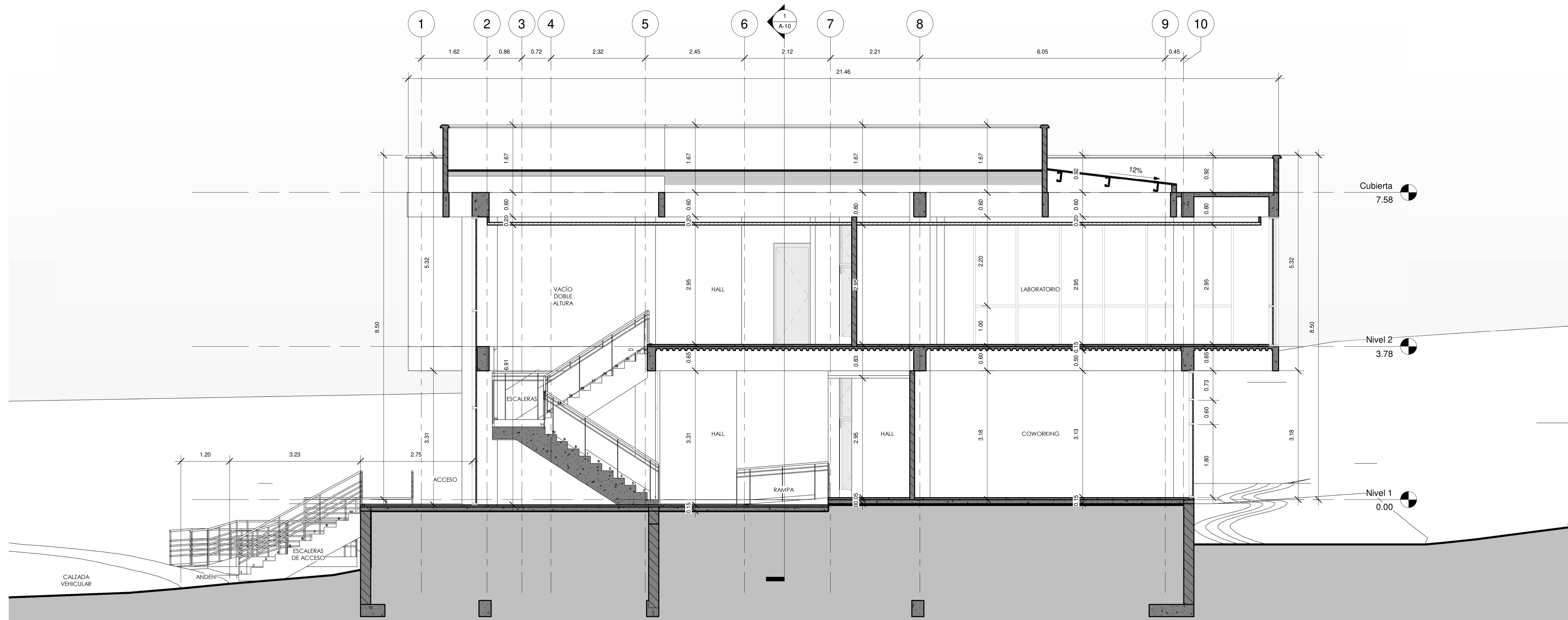
1 Corte Longitudinal A-A 1 : 50
